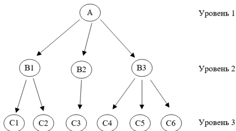
Рисунок 2.3 - Иерархическая модель данных
